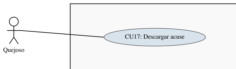
Figura 48: Diagrama de Caso de Uso CU17.
